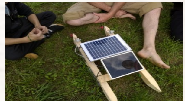
Doppelplatte mit Twin-Motor-Antrieb
